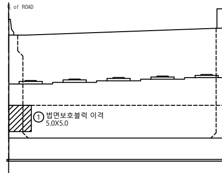
정면도
